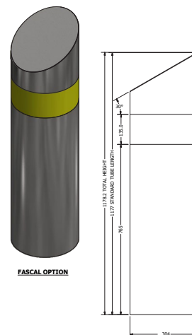
Sleeve + End Cap - 30° Mitre
